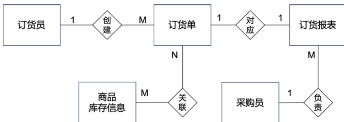
订货系统数据的 E-R 图
