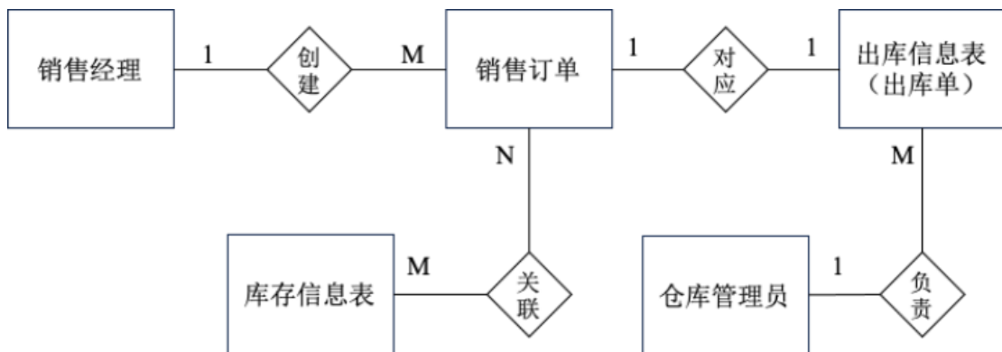
仓储系统 E-R 图
