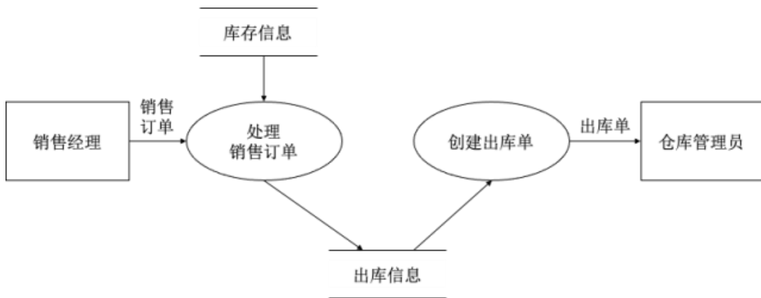
仓储系统数据流程图
